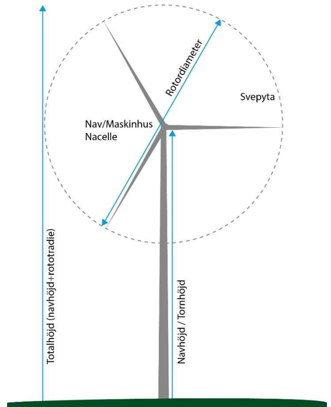
Figur 4. Principskiss över vindkraftverkets huvudsakliga beståndsdelar
