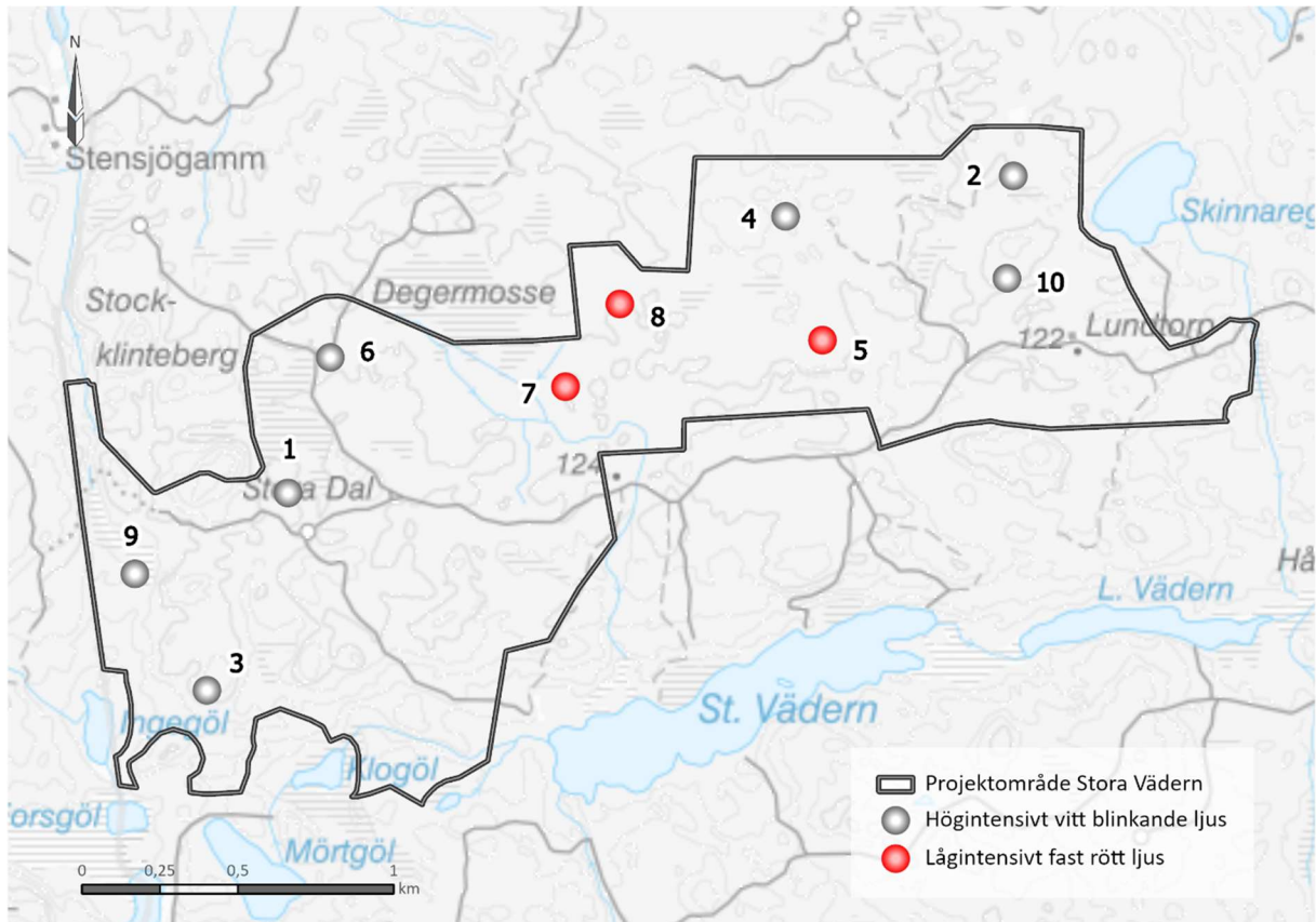
Figur 6. Exempel på placering av hinderbelysning enligt gällande föreskrifter för vindpark Stora Vädern.
