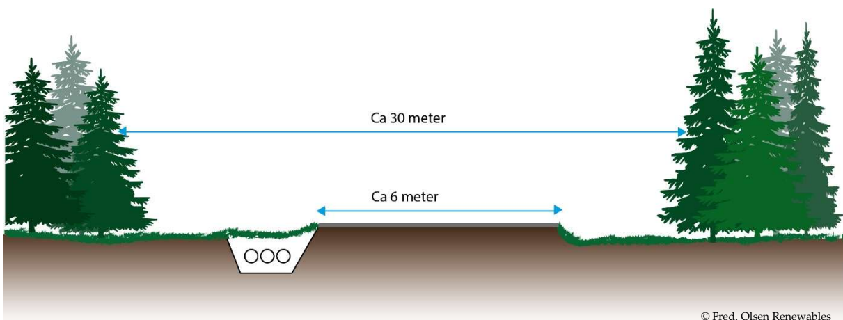
Figur 9. Principskiss vägbyggnation.
